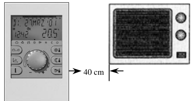
Bild 2: Mindestabstand zu anderen elektrischen Geräten
