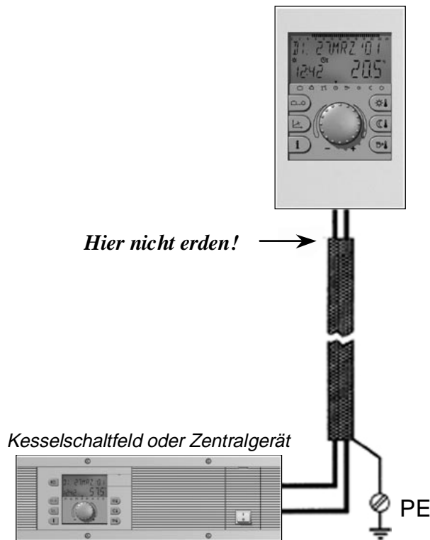
Bild 4: Einseitige Erdung der Abschirmung
