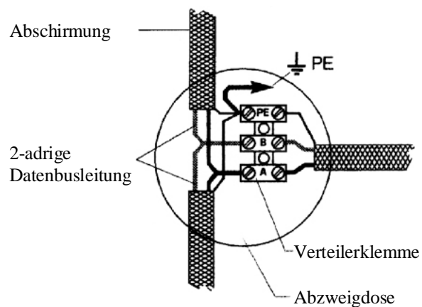
Bild 5: Erdung bei sternförmigem Datenbus
